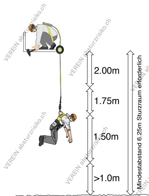
Beispiel Sturzraumbemessung
