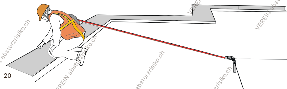
Person mit Auffanggurt und Verbindungsmittel an Anschlageinrichtung (EN 795) gesichert.
